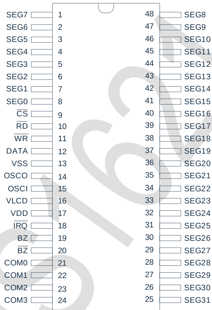
CMS1621_SSOP48
