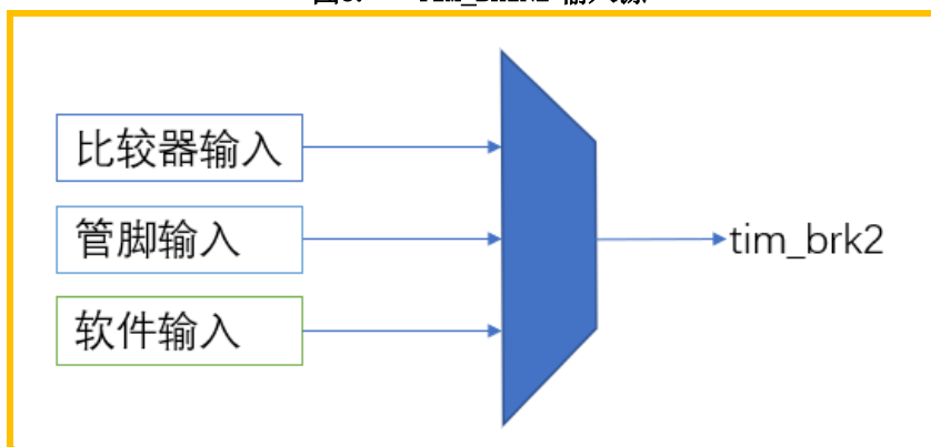
图3. TIM_BKIN2 输入源
