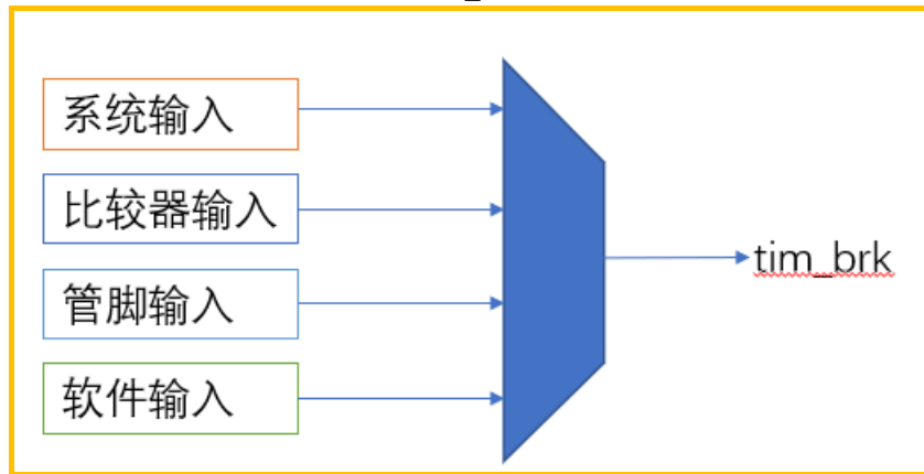
图2. TIM_BKIN 输入源
